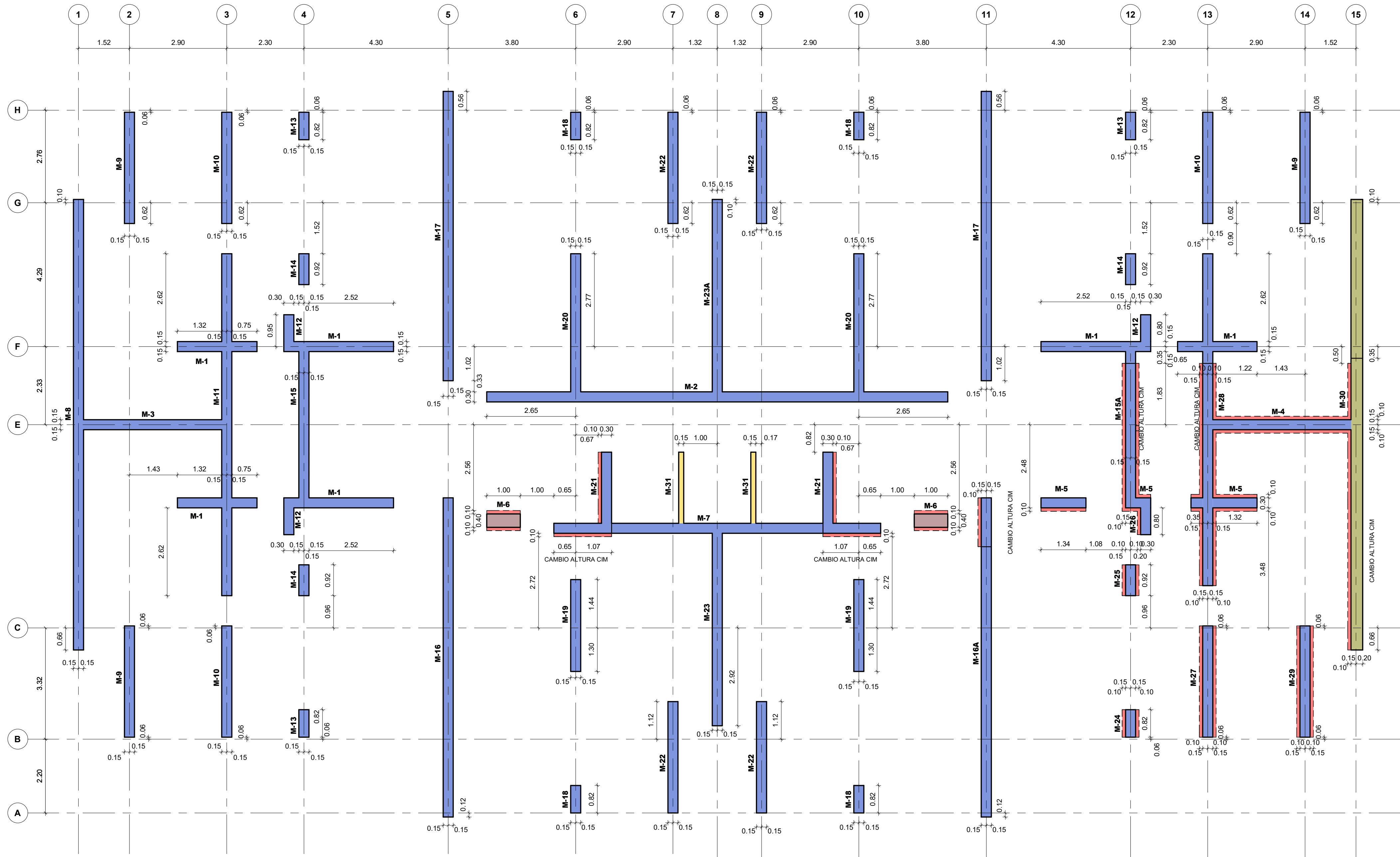
PLANTA LOCALIZACIÓN DE MUROS CIMENTACIÓN N.E -0.82 Y N.E -1.42 Escala 1 : 75
